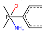
MORGAN 93
