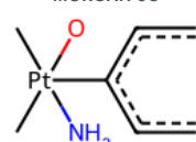
MORGAN 93
